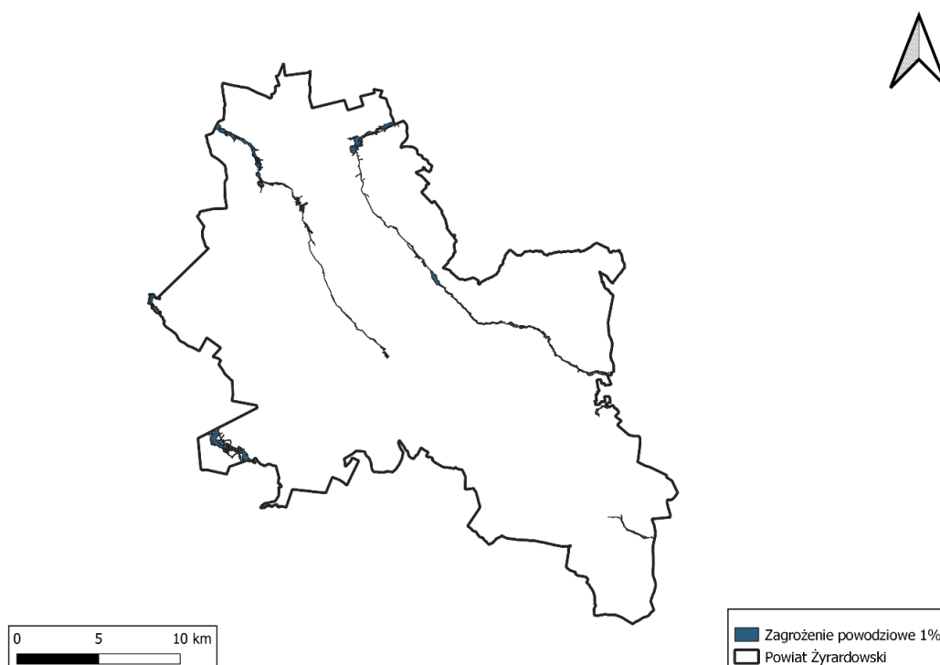
Rycina 15. Mapa zagrożenia powodziowego dla Powiatu Żyrardowskiego
