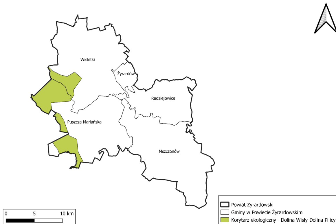
Rycina 20. Korytarz ekologiczny na terenie Powiatu Żyrardowskiego
